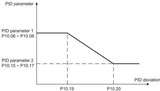
Fig 6-25 PID parameter switching
